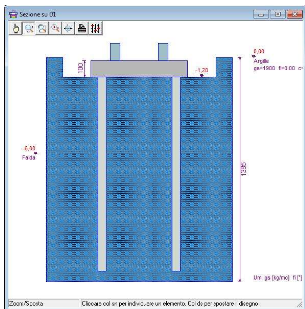
Sezione nelle condizioni iniziali predefinite
