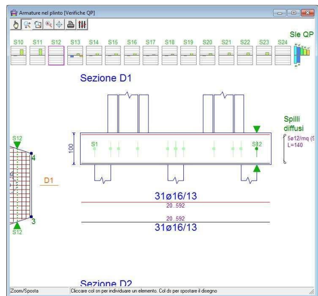
Particolare della carpenteria del plinto
