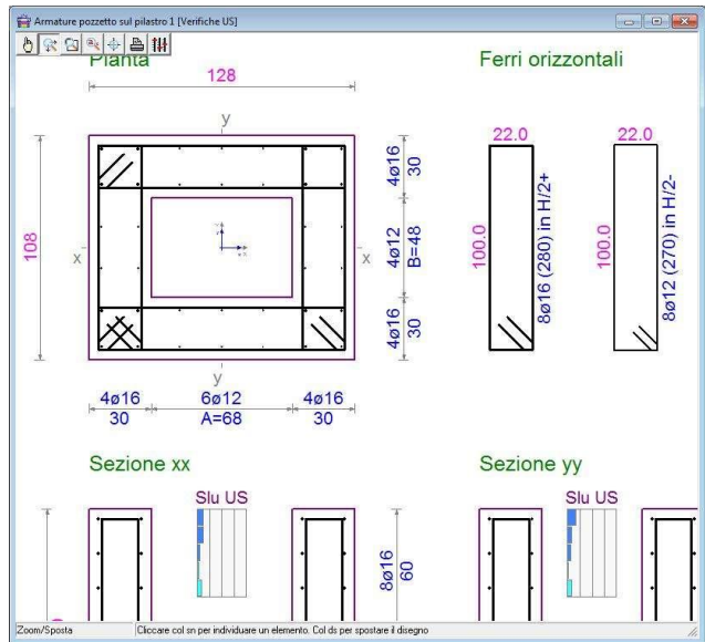
Particolare della carpenteria di un pozzetto
