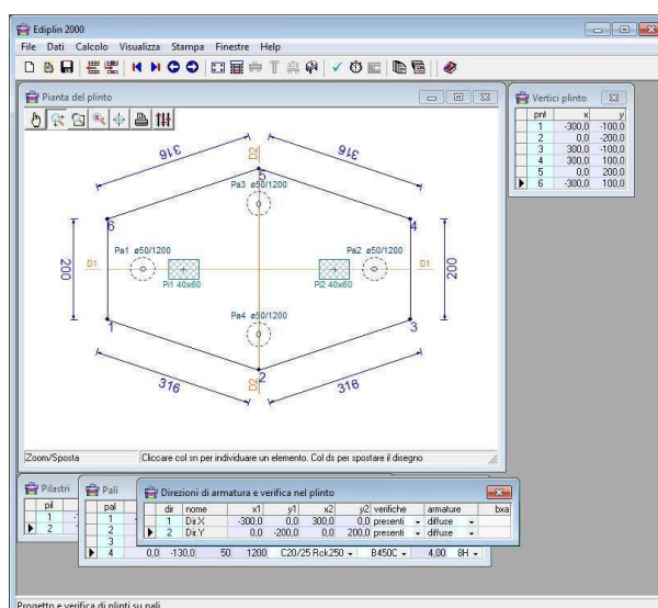
Pianta dopo la definizione dei pilastri, dei pali e delle direzioni
