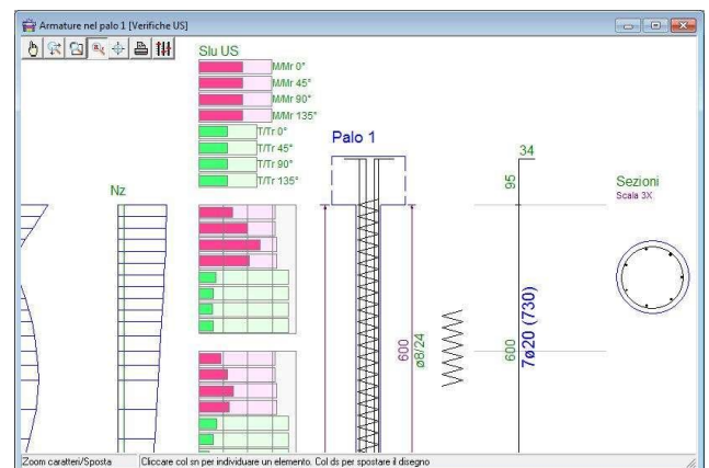
Particolare della carpenteria di un palo
