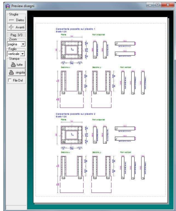
Anteprima di stampa delle carpenterie dei pali e dei pozzetti esportabili anche in Dxf o Pdf
