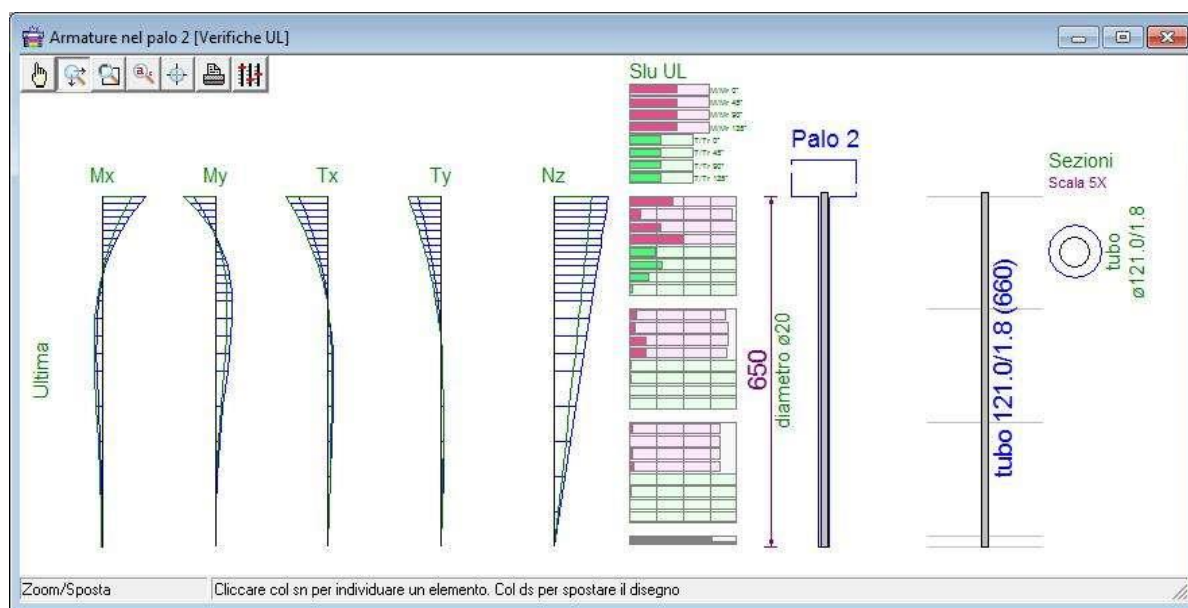
Carpenteria di un palo a tecnologia tubfix
