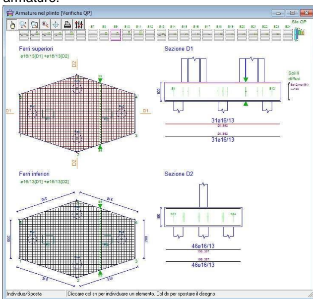
Vista della carpenteria del plinto
