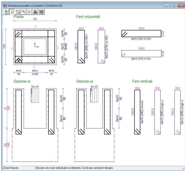
Vista della carpenteria di un pozzetto
