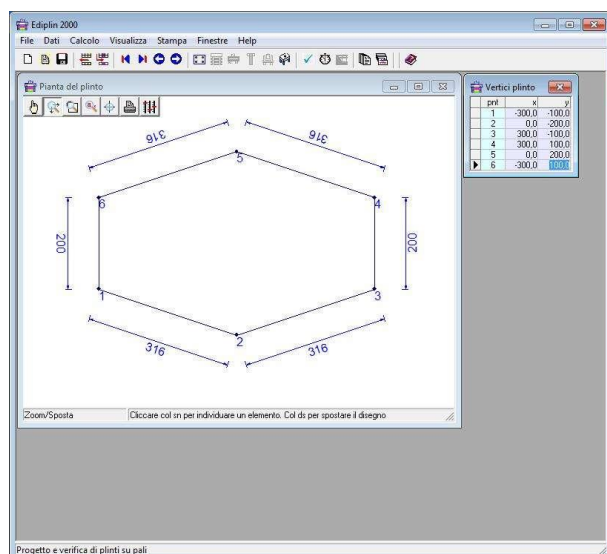
Pianta dopo la definizione dei sei vertici
