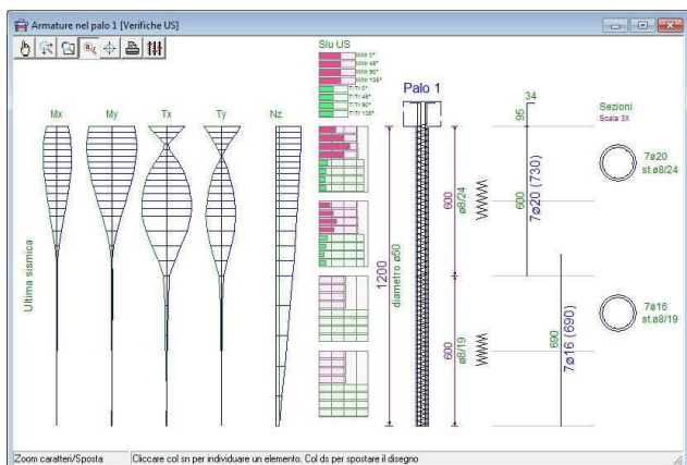
Vista della carpenteria di un palo
