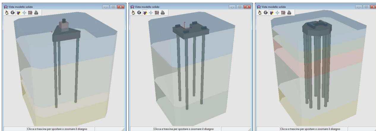
Vista solida di plinti definiti col programma
