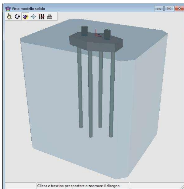
Vista solida tridimensionale corrispondente
