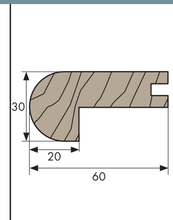
PROFILO PER SCALE STONATO 60 X 30 STAIR PROFILE - ROUNDED TREPPENKANTE ABGERUNDET
