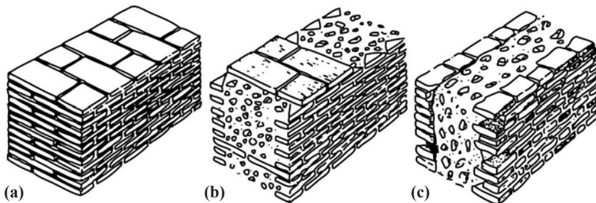
Figura 1.1. (a) muratura regolare; (b) muratura a secco con elementi trasversali di collegamento; (c) muratura a secco (Drysdale et al., 1999)
