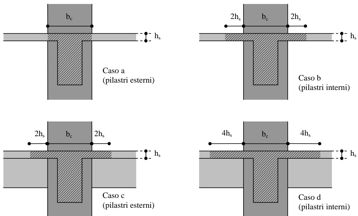
Figura 7.4.2 – Larghezza collaborante delle travi.
