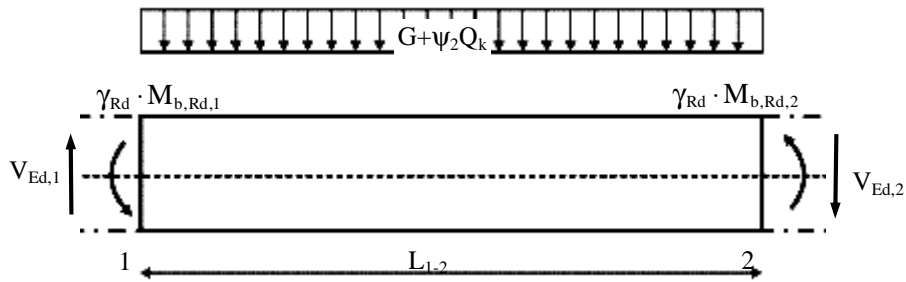
Figura 7.4.1 – Determinazione delle forze di taglio di calcolo per le travi.
