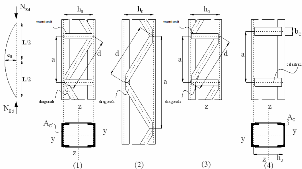
Figura C4.2.7 - Aste composte costituite da due correnti uguali
