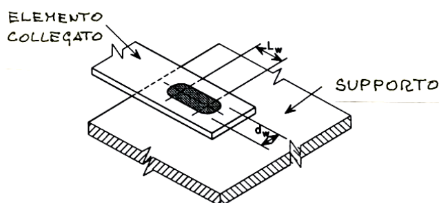
Figura C4.2.36 – Saldature oblunghe a bottone
