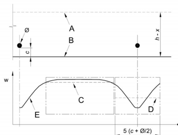
Fig. C4.1.10 Spaziatura tra le barre.
