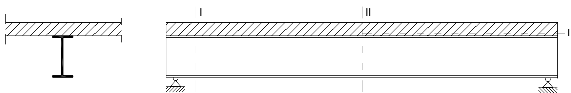
Figura C4.3.5 – Trave d'acciaio con soletta collaborante
