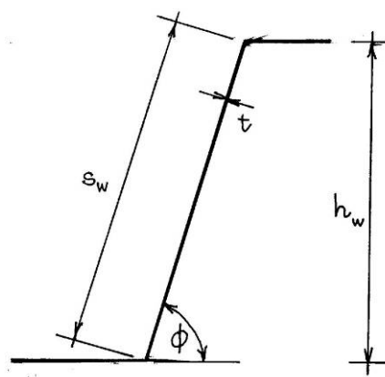
Figura C4.2.33 – Anime di profili sottili
