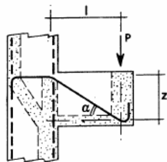
Figura C4.1.8 Esempi di modello a puntoni e tiranti con tirante obliquo per mensole tozze
