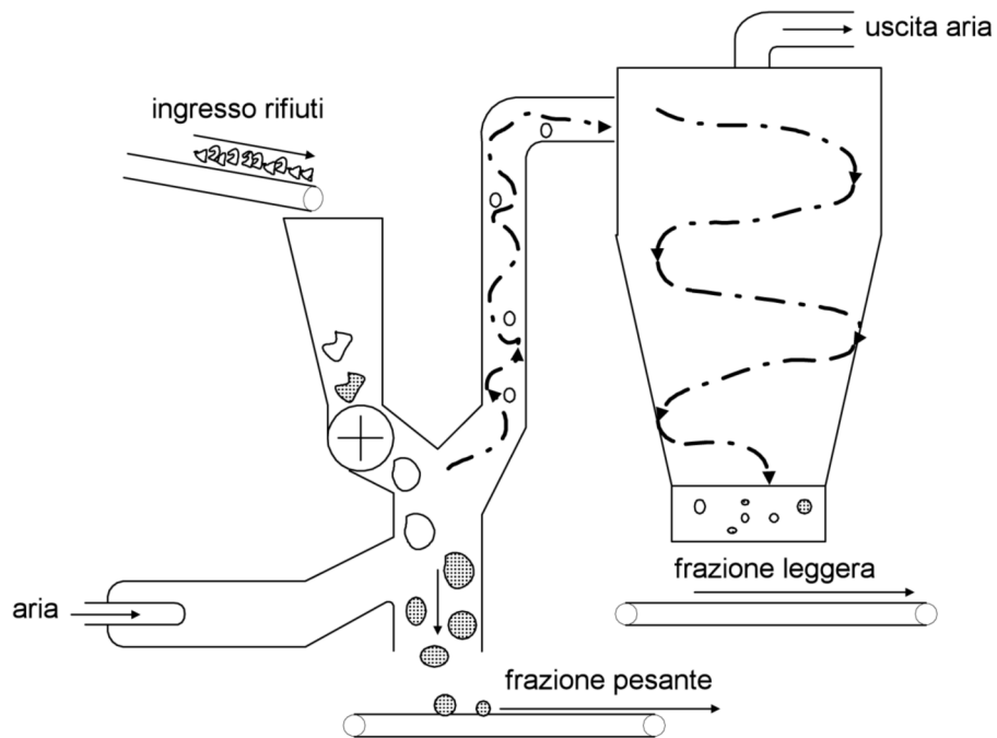
Figura A7 Classificatore aeraulico a coltello
