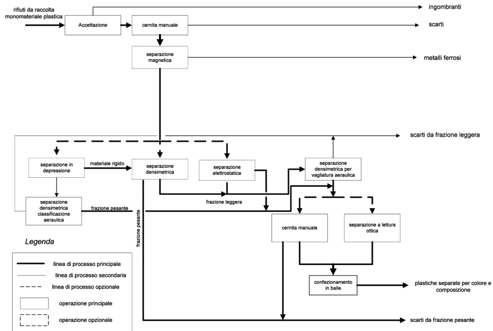
Figura A21 Schema di principio di una linea di selezione di vetro da raccolta monomateriale
