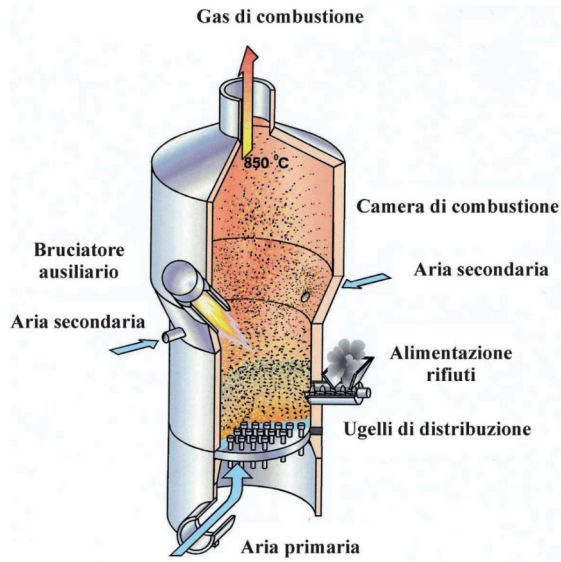
Figura A48 Schema di funzionamento del combustore a letto fluido circolante
