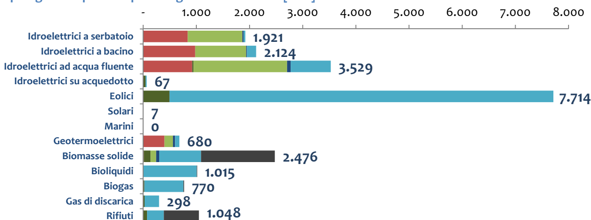
Figura 6. Potenza complessiva degli impianti qualificati e in esercizio al 31 dicembre 2012, suddivisi per tipologia di impianto e per categoria di intervento [MW].
