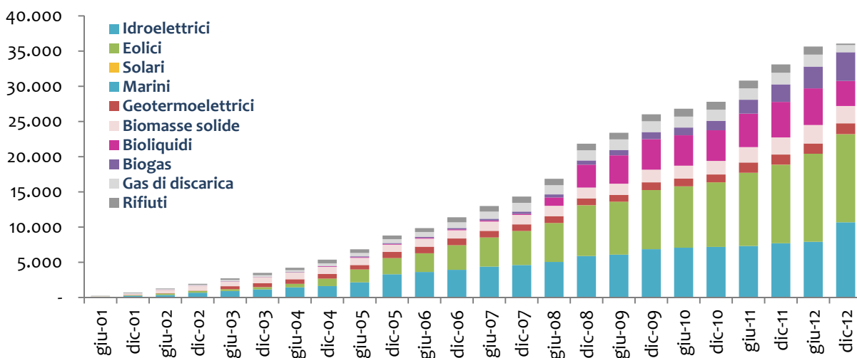
Figura 20. Andamento per semestre dell'energia incentivabile degli impianti qualificati e entrati in esercizio. Suddivisione per tipologia di impianto [GWh].
