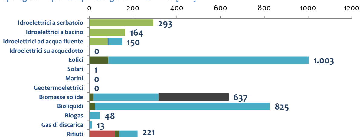
Figura 10. Potenza complessiva degli impianti qualificati a progetto al 31 dicembre 2012, suddivisi per tipologia di impianto e per categoria di intervento [MW]
