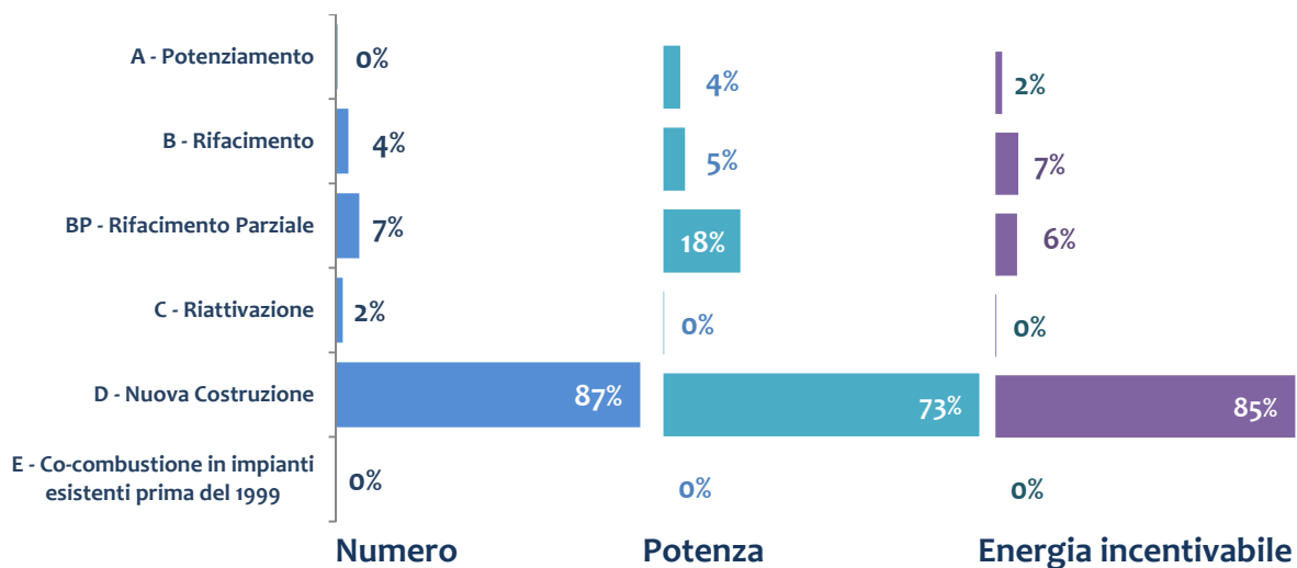
Figura 4. Impianti qualificati a progetto al 31 dicembre 2012. Suddivisione per categoria di intervento.
