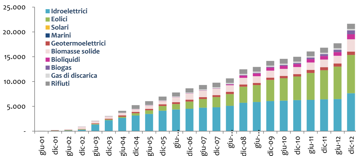
Figura 19. Andamento per semestre della potenza degli impianti qualificati e entrati in esercizio. Suddivisione per categoria di intervento [MW].
