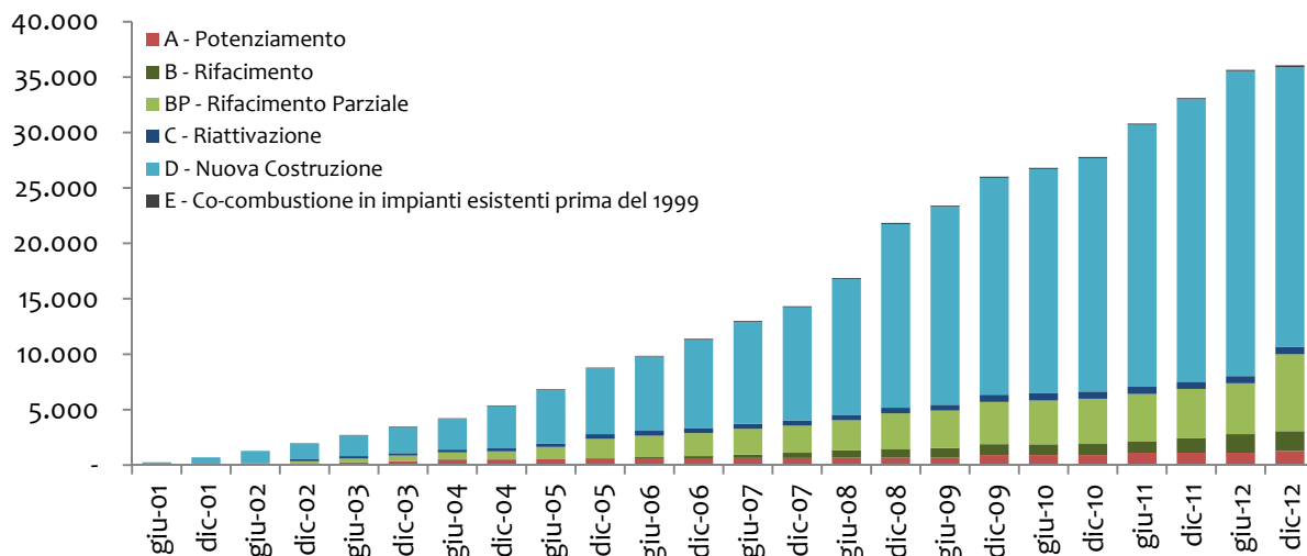
Figura 21. Andamento per semestre dell'energia incentivabile degli impianti qualificati e entrati in esercizio. Suddivisione per categoria di intervento [GWh].
