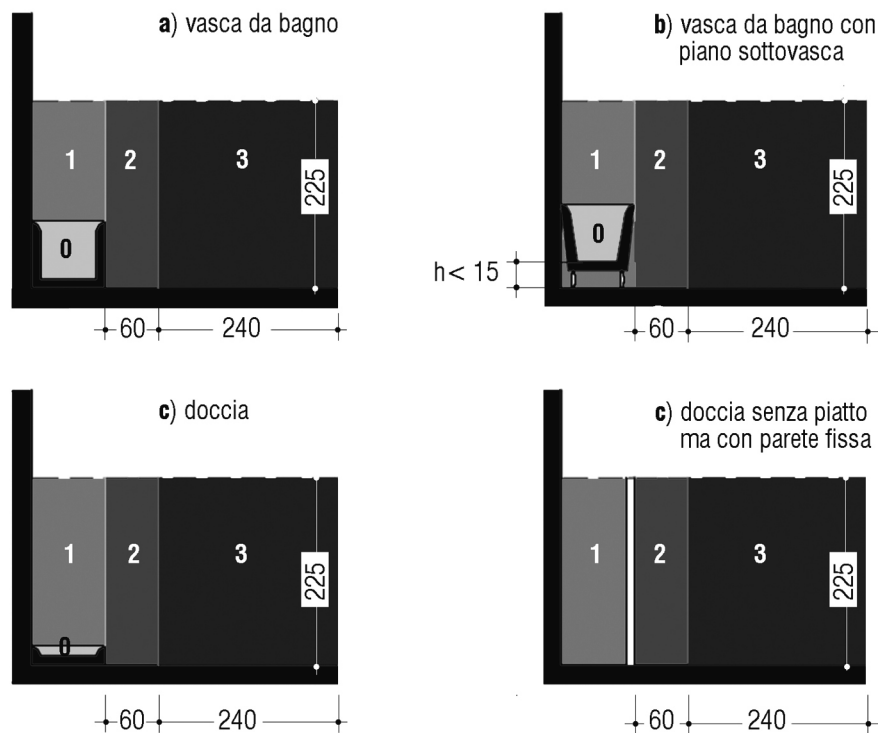
2.1 Zone dei bagni -sezioni- (NORMA CEI 64-8/7 VI ed.). (Misure in cm)
