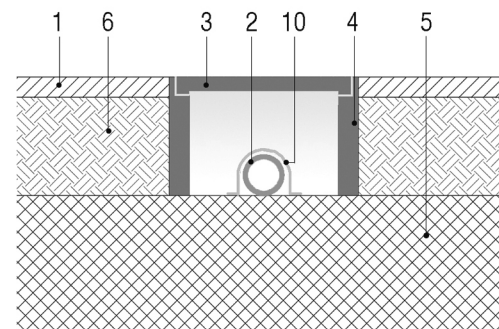
2.2 Posa interrata della tubazione entro apposita entro apposita canaletta all'interno di un manufatto
