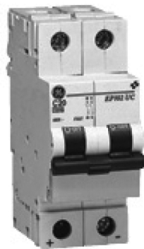
1.2 Esempio di sezionatore 1F+N
