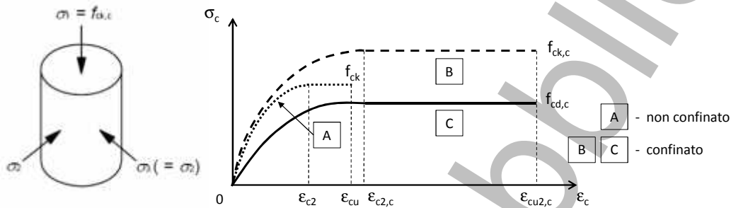
Fig. 4.1.2 – Modelli \sigma - \varepsilon per il calcestruzzo confinato
