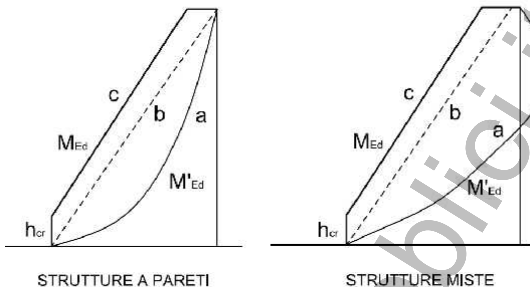
Fig. 7.4.4 – Traslazione del diagramma dei momenti flettenti per strutture a pareti e strutture miste
