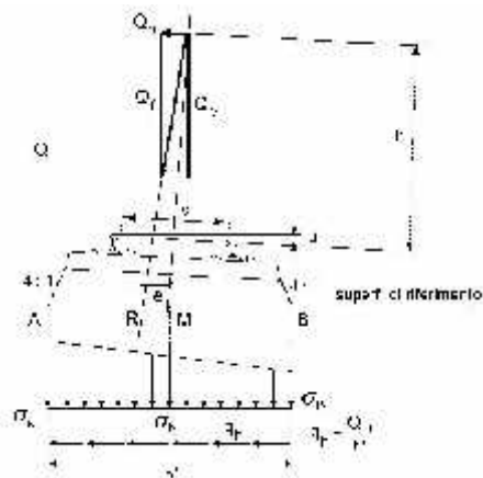
Fig. 5.2.6 - Distribuzione trasversale in curva delle azioni per mezzo delle traverse e del ballast. In figura, Q_1 rappresenta la forza centrifuga definita al successivo §5.2.2.3.1
