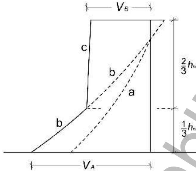
Fig. 7.4.5 – Diagramma di involucro delle forze di taglio nelle pareti di strutture miste
