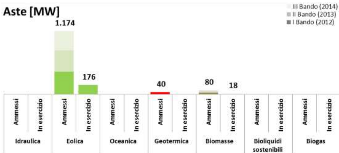
Figura 3 Potenza degli impianti che al 31/12/2014 risultano ammessi in posizione utile nei registri o aggiudicatari di procedure d'asta, con indicazione della quotaparte di essi che risultano in esercizio al 31/12/2014, per specifica tecnologia e schema di incentivazione (Registri, Aste, Rifacimenti).
