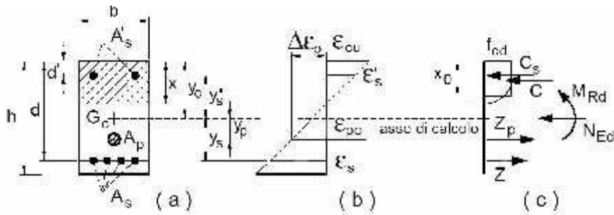
Fig. 4.1.4 – Sezione
