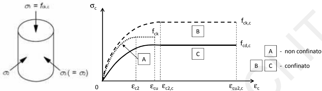
Fig. 4.1.2 Modelli \sigma - \varepsilon per calcestruzzo confinato
