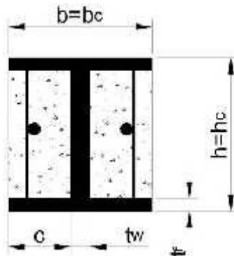
Fig. 7.6.1 - Rapporti dimensionali
