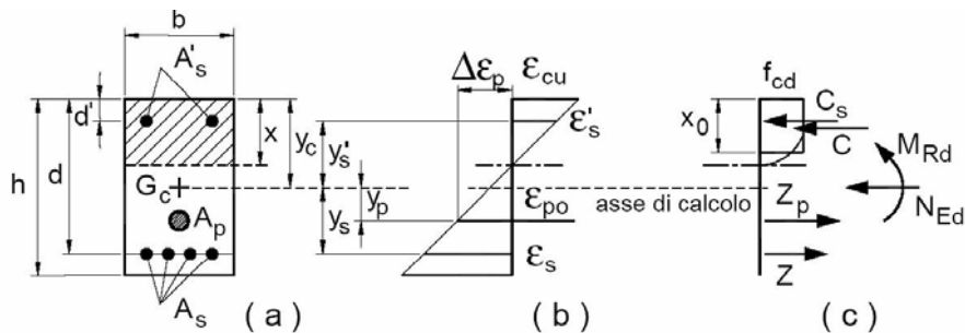
Fig. 4.1.4 – Sezione pressoinflessa
