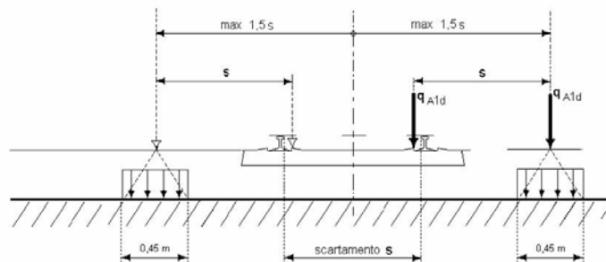
Fig. 5.2.12 - Caso 1
