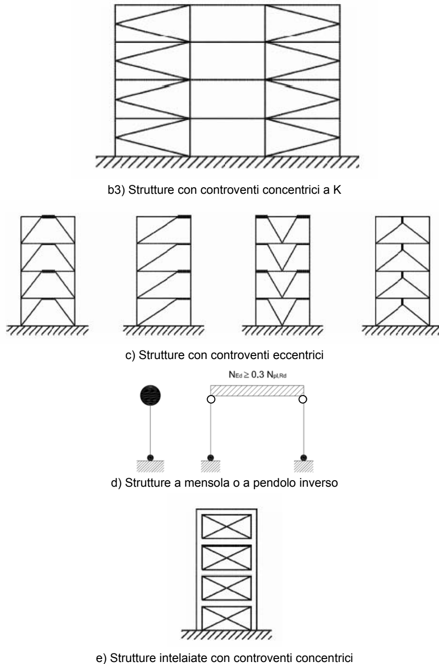
Fig. 7.5.1. - Tipologie strutturali
