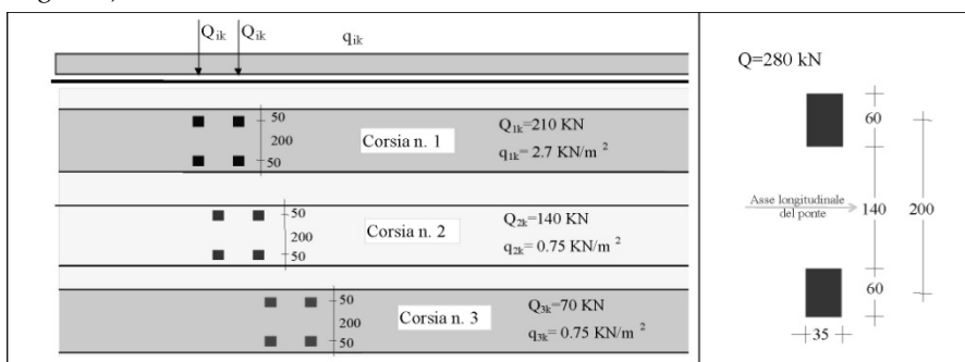
Fig. 5.1.4 - Modello di carico di fatica 1
