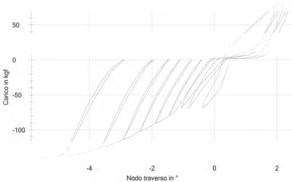
Figura 3-117 Curva carico – inclinazione trasverso al nodo
