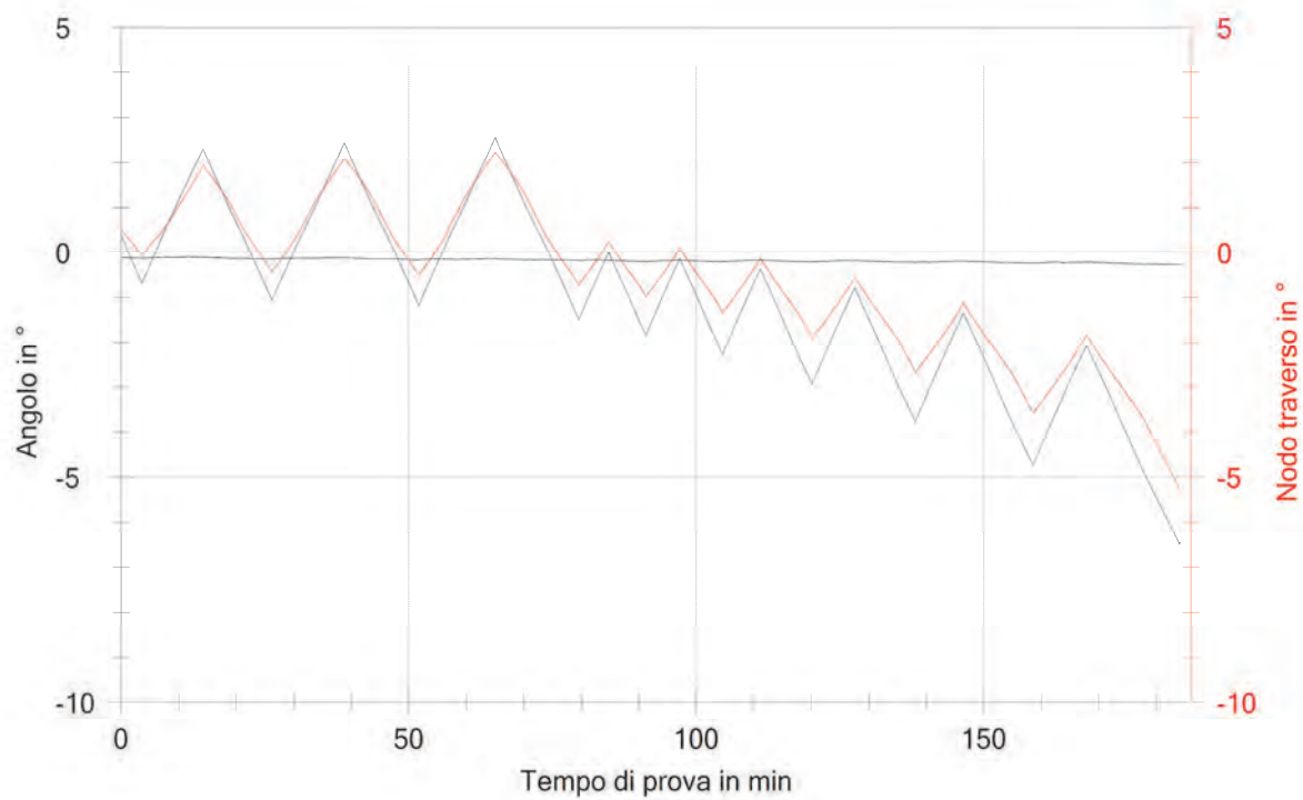
Figura 3-112 Inclinazione nodo trasverso, nodo libero e nodo montante nel tempo
