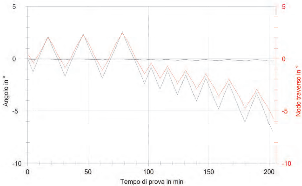
Figura 3-118 Inclinazione nodo trasverso, nodo libero e nodo montante nel tempo
