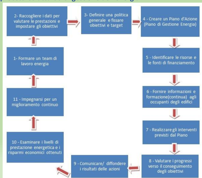
Figura 5.6 – Schema di processi strutturati di gestione dell'energia
