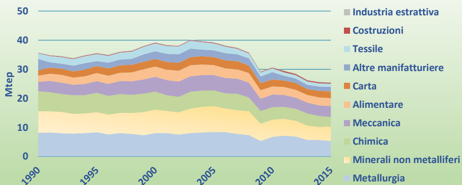
Figura 2.10 – Consumo energetico nell'industria per comparto produttivo (Mtep), anni 1990-2015
