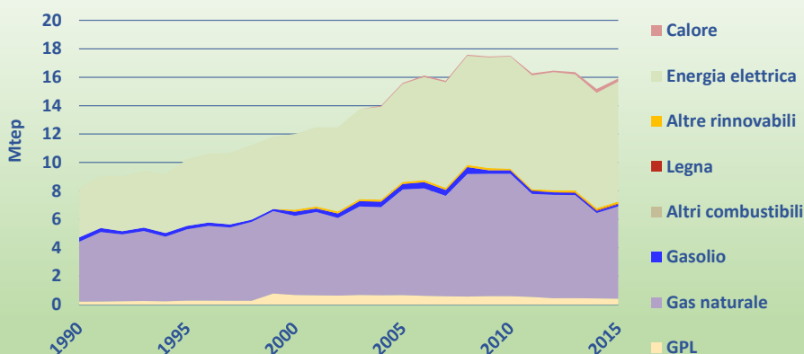
Figura 2.15 – Consumo energetico nel settore non residenziale per fonte (Mtep), anni 1990-2015
