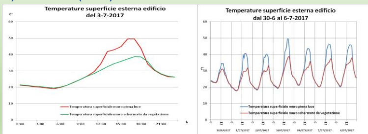
Figura 5.4 – Misurazione della temperatura della superficie esterna dell'edificio, giornaliera (sinistra) e settimanale (destra)
