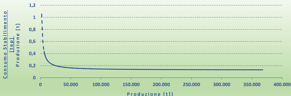
Figura 4.7 – Indice di prestazione generale di stabilimento per la produzione di ceramica
