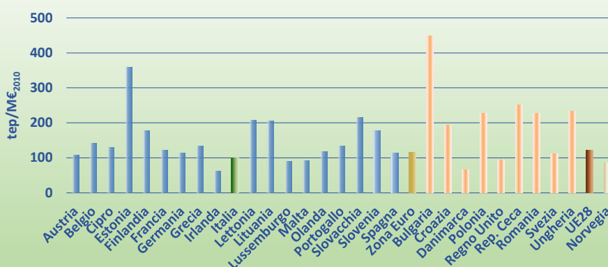
Figura 2.21 – Intensità energetica primaria dei Paesi UE28 (tep/M€ 2010 ), anno 2015
