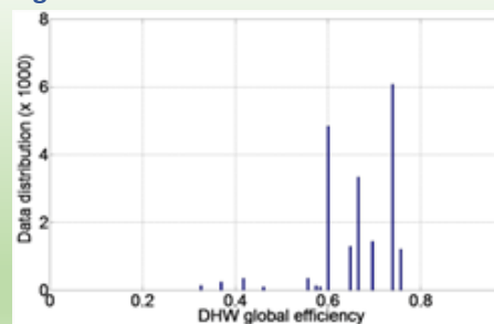
Figura 2.14 – Rendimenti medi ACS
