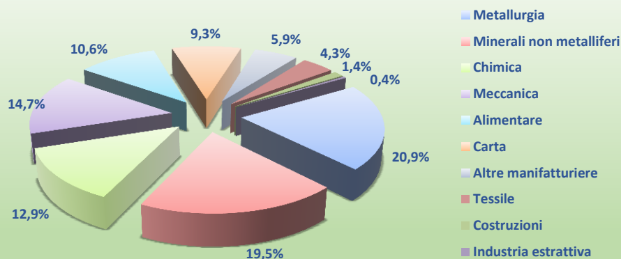
Figura 2.11 – Consumo energetico nell'industria per comparto produttivo (%), anno 2015
