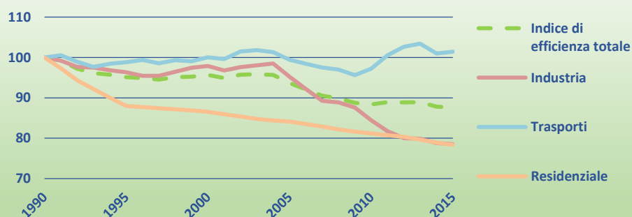
Figura 2.26 – Indice di efficienza energetica ODEX (1990=100), anni 1990-2015
