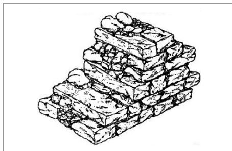
Sezione muraria con abbondante presenza di elementi di collegamento (diàtoni) tra i due paramenti.
