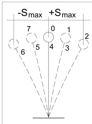
Figura 10.1. Sistema elementare con 1 massa
