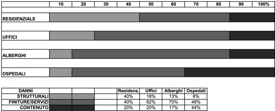
Figura 13.1. Tipologie di danni causati da terremoti
