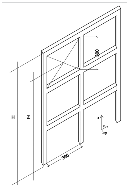
Figura 12.2. Modello del tamponamento sull'ossatura in calcestruzzo armato
