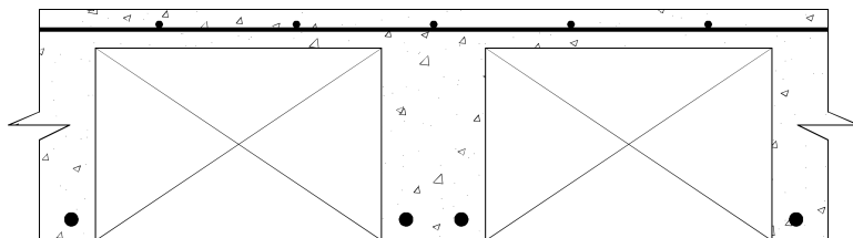
Figura 9.2. Solaio misto.
