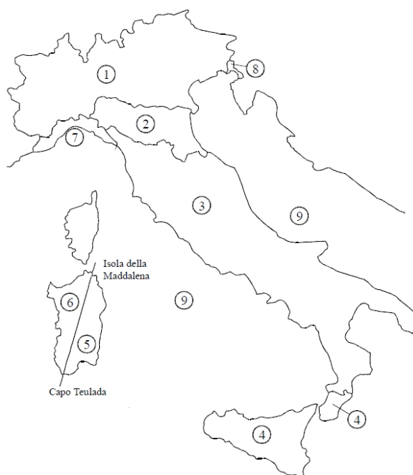
Figura 6.1. Mappa delle zone in cui è suddiviso il territorio italiano (§ 3.3.1 delle NTC 2018).
