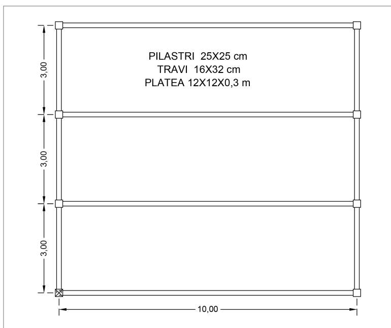
Figura 6.1a). Pianta della struttura
