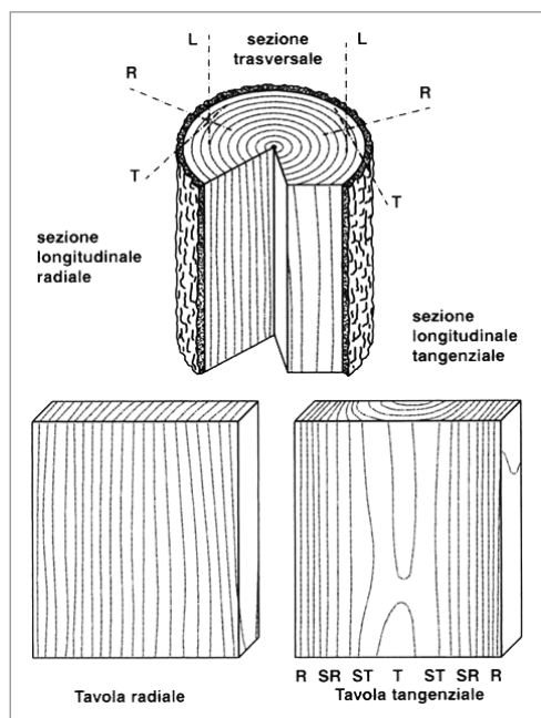
Figura 3.1. Costituzione del tronco
