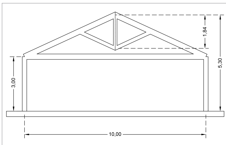
Figura 6.1b). Prospetto della struttura
