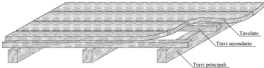
Figura 13.2. Solaio composto
