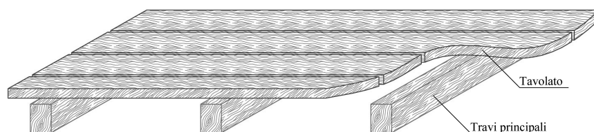
Figura 13.1. Solaio semplice
