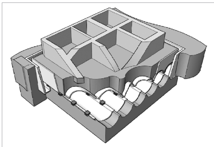
Figura 6.1. Struttura di isolamento sismico per edifici esistenti: spaccato assonometrico
