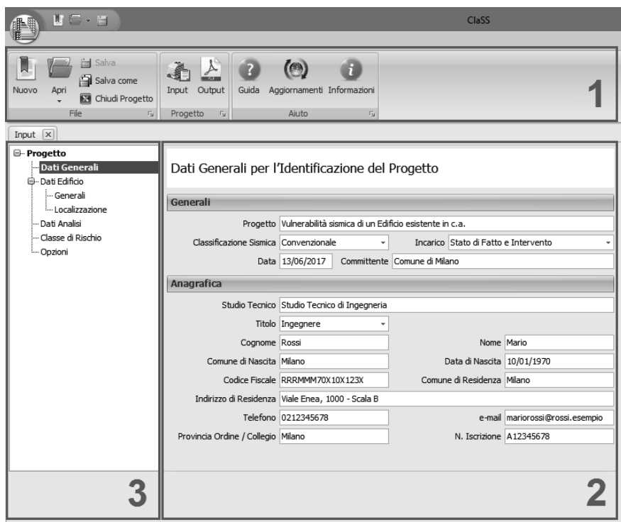
Figura 4.1. Interfaccia Utente
