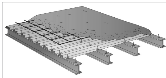
Figura 19.1. Solaio in lamiera grecata e travi in acciaio
