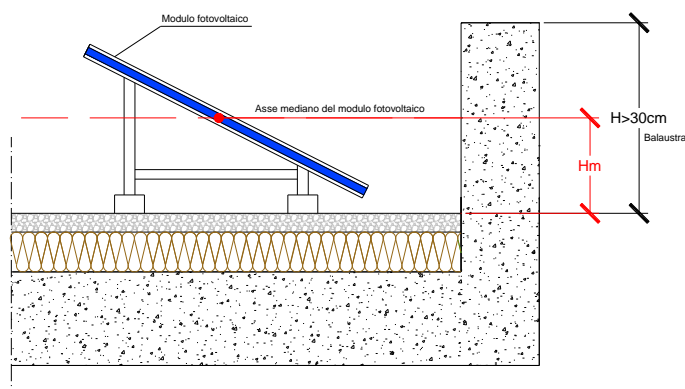
Figura 3 – Caso 2, H > 30\text{cm} - Schema esemplificativo di un'installazione idonea alla classificazione dell'impianto fotovoltaico nella categoria "su edifici"
