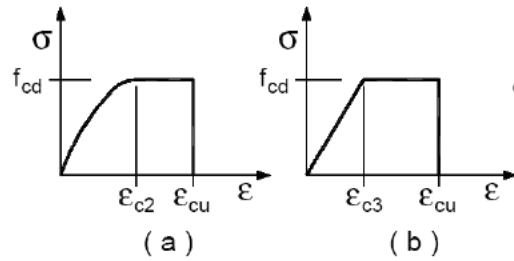
Figura C4.1.13 -Modelli \sigma - \epsilon per il calcestruzzo di aggregati leggeri
