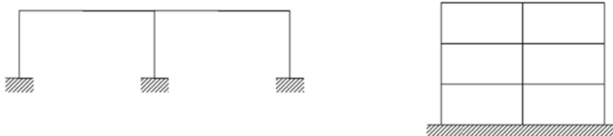
Figura C7.4.4 - Strutture a telaio con collegamenti monolitici
