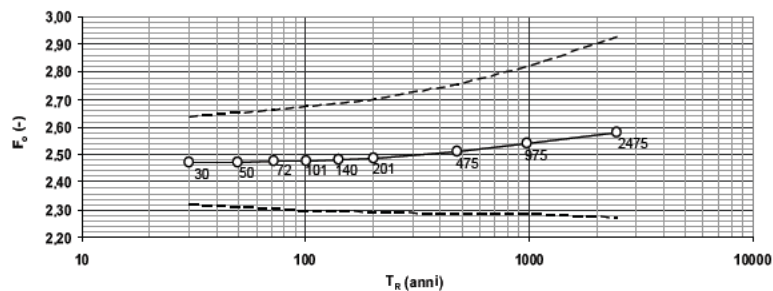
Figura C3.2.1 b – Variabilità di F_0 con T_R : andamento medio sul territorio nazionale ed intervallo di confidenza al 95%
