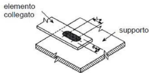
Figura C4.2.36 – Saldature oblunghine a bottone
