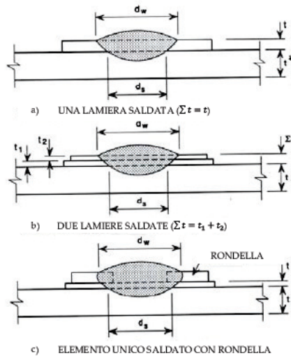
Figura C4.2.35 – Saldature a bottone
