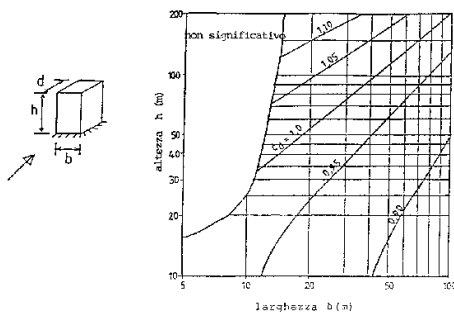
Fig. 7.10. (b) - Edifici a struttura in acciaio
