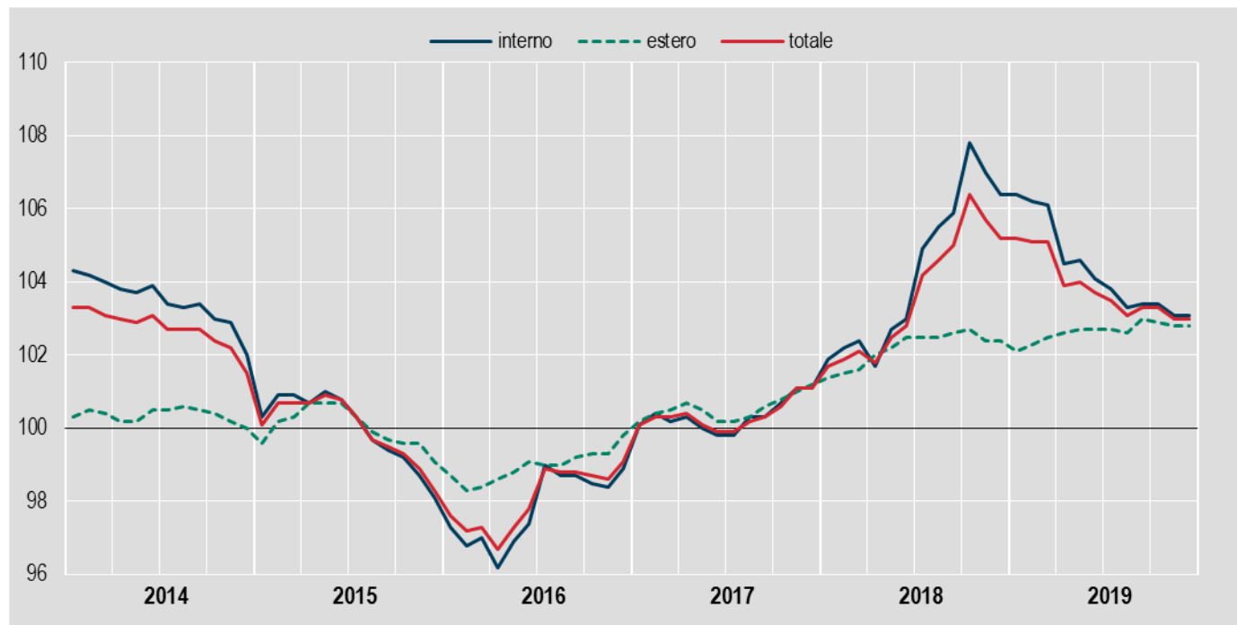
FIGURA 1. NUMERI INDICE DEI PREZZI ALLA PRODUZIONE DELL'INDUSTRIA PER MERCATO DI RIFERIMENTO Gennaio 2014 – dicembre 2019 (base 2015=100)
