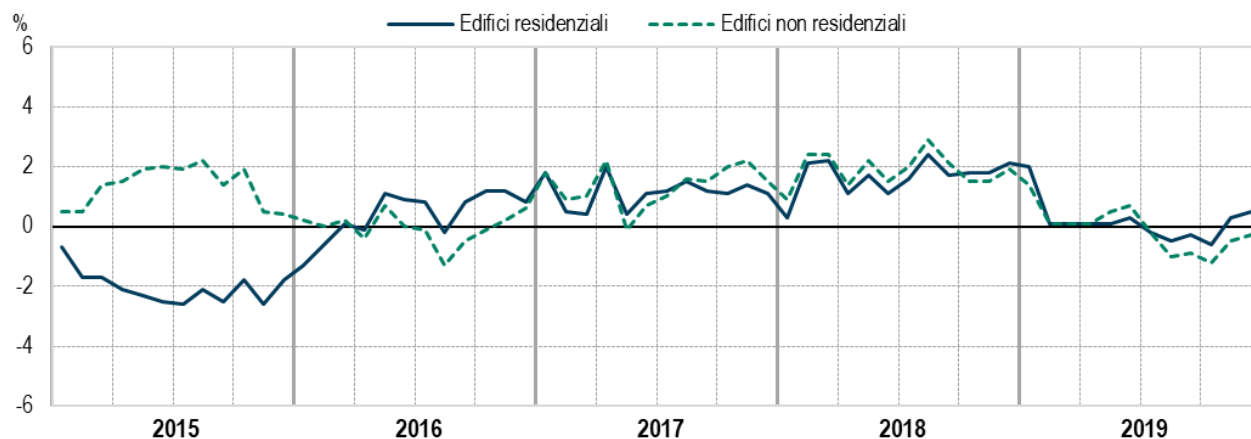
FIGURA 6. PREZZI ALLA PRODUZIONE DELLE COSTRUZIONI. EDIFICI RESIDENZIALI E NON RESIDENZIALI Gennaio 2015 – dicembre 2019, variazioni percentuali tendenziali (base 2015=100)
