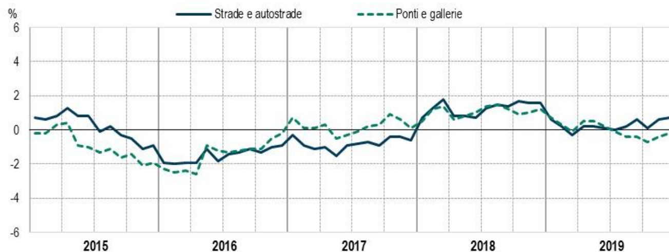
FIGURA 10. PREZZI ALLA PRODUZIONE DELLE COSTRUZIONI. STRADE E AUTOSTRADE, PONTI E GALLERIE
