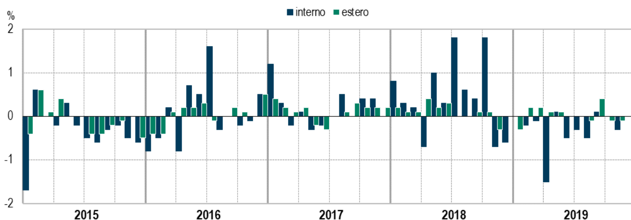
FIGURA 2. PREZZI ALLA PRODUZIONE DELL'INDUSTRIA, VARIAZIONI PERCENTUALI CONGIUNTURALI Gennaio 2015 – dicembre 2019 (base 2015=100)
