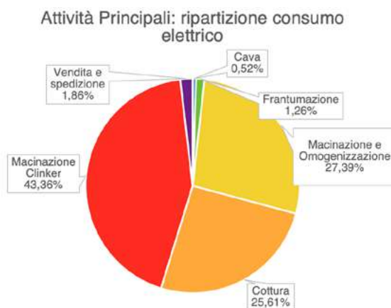
Figura 12 – Ripartizione dei consumi medi elettrici per la produzione di cemento grigio tra le differenti fasi del processo produttivo all'interno delle attività principali
