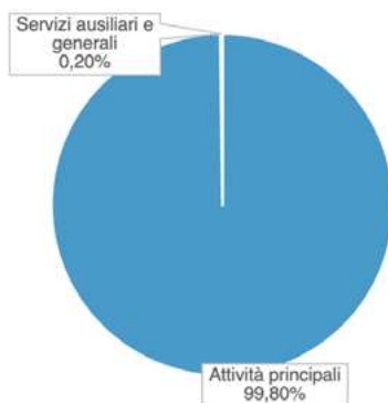
Figura 10 – Ripartizione dei consumi termici per la produzione di cemento grigio tra le differenti aree funzionali
