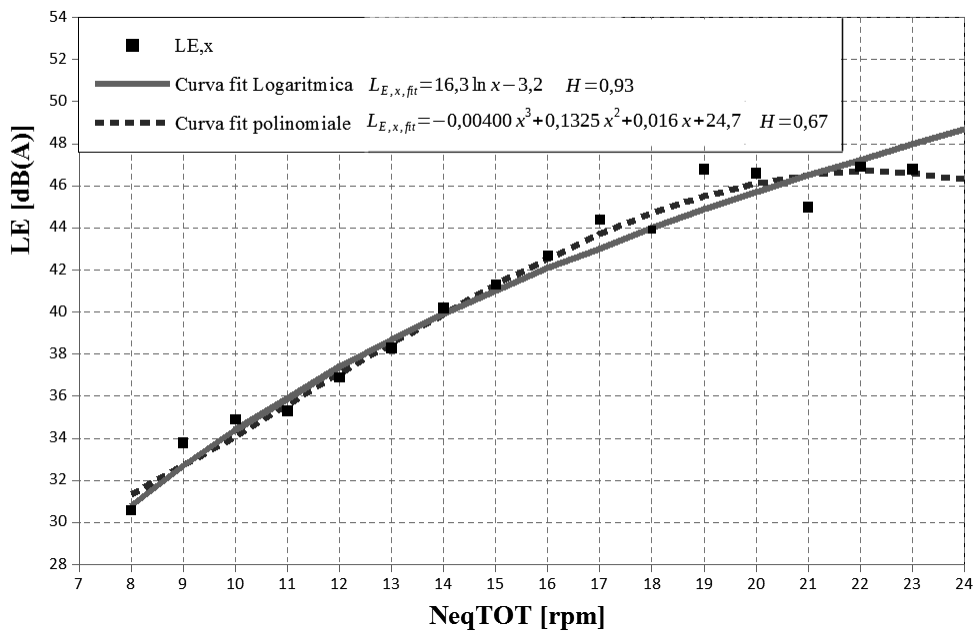
Fig. 8: Esempio di curve di fit ottenute con il metodo dei minimi quadrati applicato ai valori di L_{E,x} ricavati con la procedura di calcolo.
